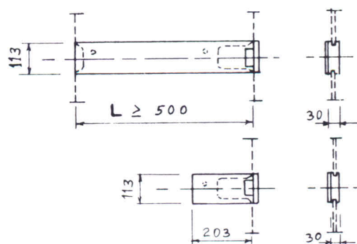
MANIGLIONE CON BOCCHETTA ELETTRICA "EFFE FR."
